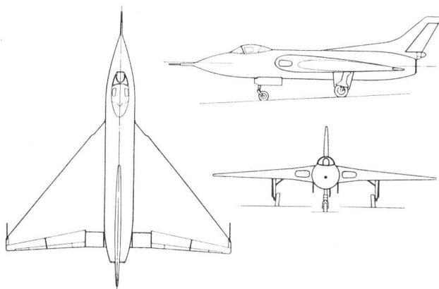
Uebersichtszeichnung des DELTA-Flugzeuges AVRO 707-A Links: Draufsicht; oben: Seitenansicht; unten: Vorderansicht. (Siehe Umschlagseite dieser Nummer)
