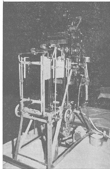
Aus der Sowjetunion herausgeschmuggelt und im Westen wieder montiert: eine von den EChB-Mitgliedern selbst gebastelte Offset-Druckmaschine für den Untergrundverlag Christianin. Der Motor stammt aus einer Waschmaschine. Das erste Modell lief noch mit einer Fleischwolf-Kurbel im Handantrieb. Die EChB-Gemeinden verbreiten in der UdSSR religiöse Literatur; dafür verfolgt sie das KGB.
