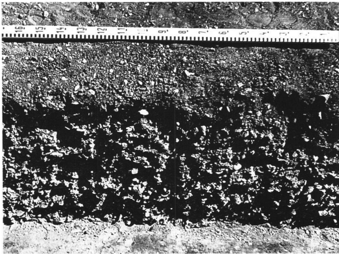
Abb. 46 Ausschnitt der beidseits des Ofens festgestellten Schlackenschicht. Der Schlackenanstoss war beim Verhütten der Doggererze in Berslingen gross.
