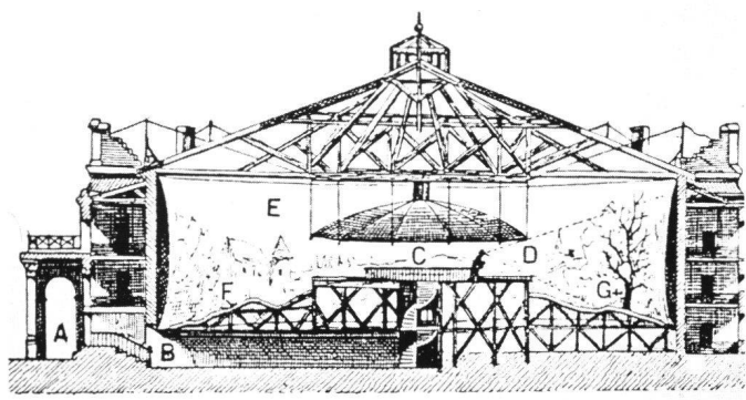
Abb. 3 Schnitt durch die übliche Panorama-Konstruktion (aus: ST. OETTERMANN, Das Panorama ).
