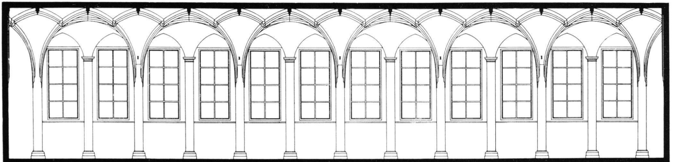
Abb. 2 Basel, Spießhof, Gewölbesaal, Aufriß der Fensterwand
