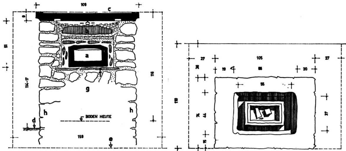
Abb. 6. – Blockaltar der Kirche St. Lorenz bei Paspels (nach Entfernung der barocken, seitlichen Anmauerungen): links Aufriss, rechts Querschnitt auf der Höhe des Sepulcrums:
