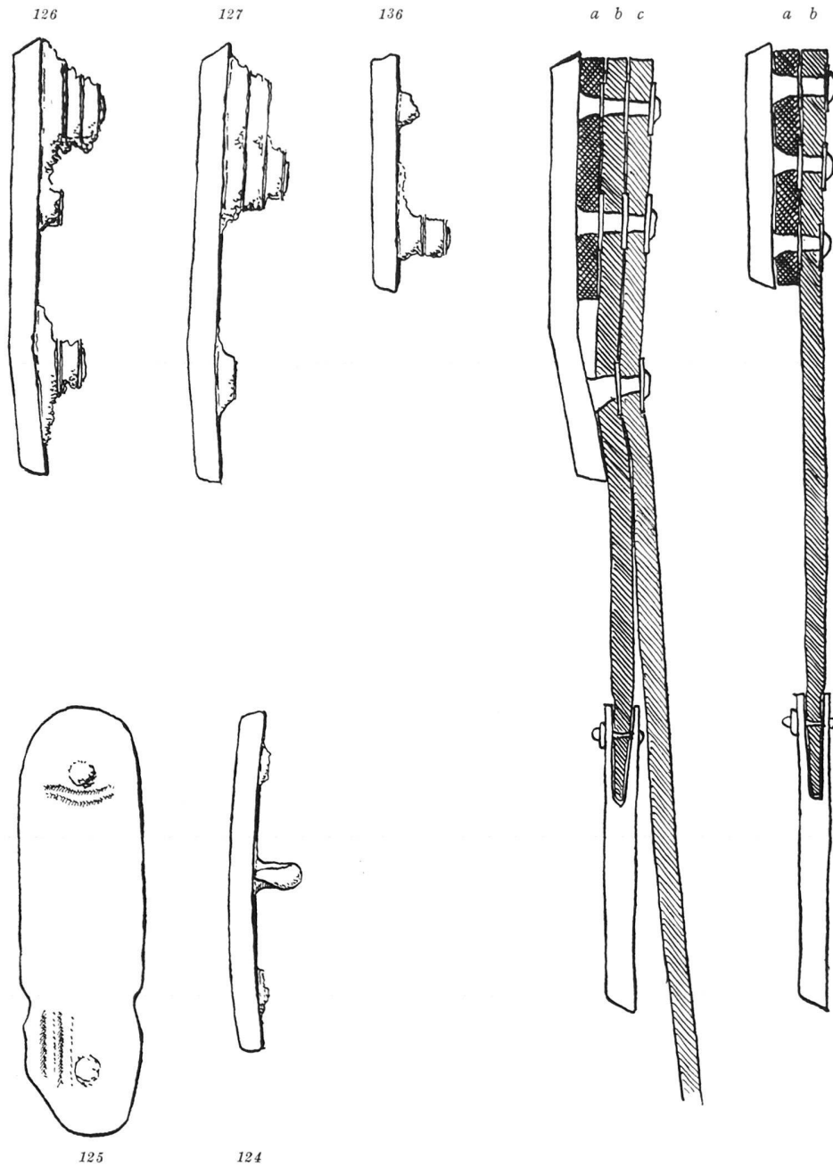
Abb. 13. Befestigungsarten der Vertikalbeschläge 126, 127. Bei Beschläg 125 noch Lederspuren. Bei Beschläg 124 ist der mittlere Ösenniet erhalten. – Rechts : Rekonstruktion der Befestigung: a Gürtelriemen, b Nebenriemen, c Wehrgehänge (nur bei den drei Vertikalbeschlägen).
