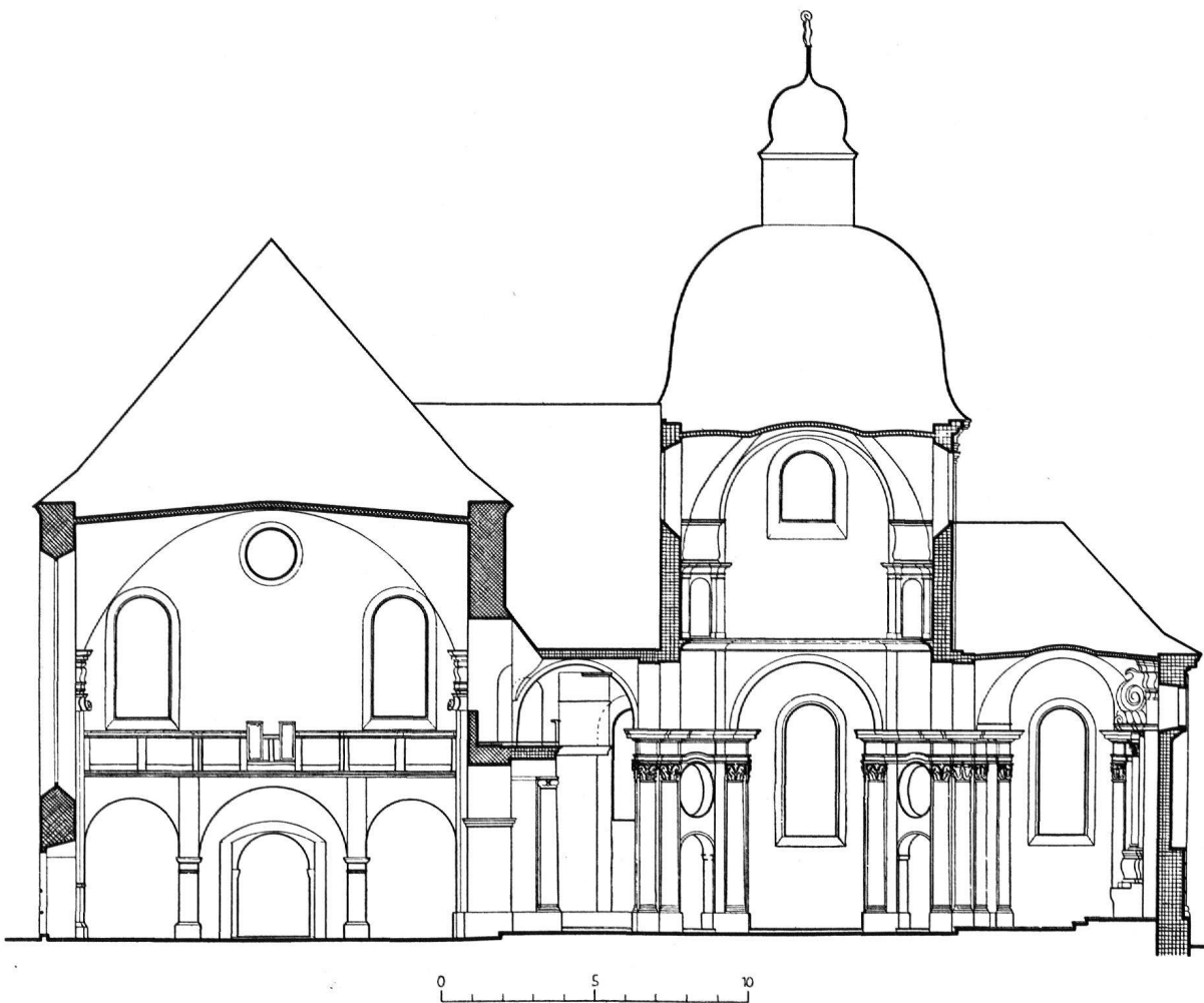
Abb. 2. Fischingen, Kirche und Iddakapelle, Schnitt von Süden nach Norden mit Blick auf Westpartien (Aufnahme Oskar Schaub)
