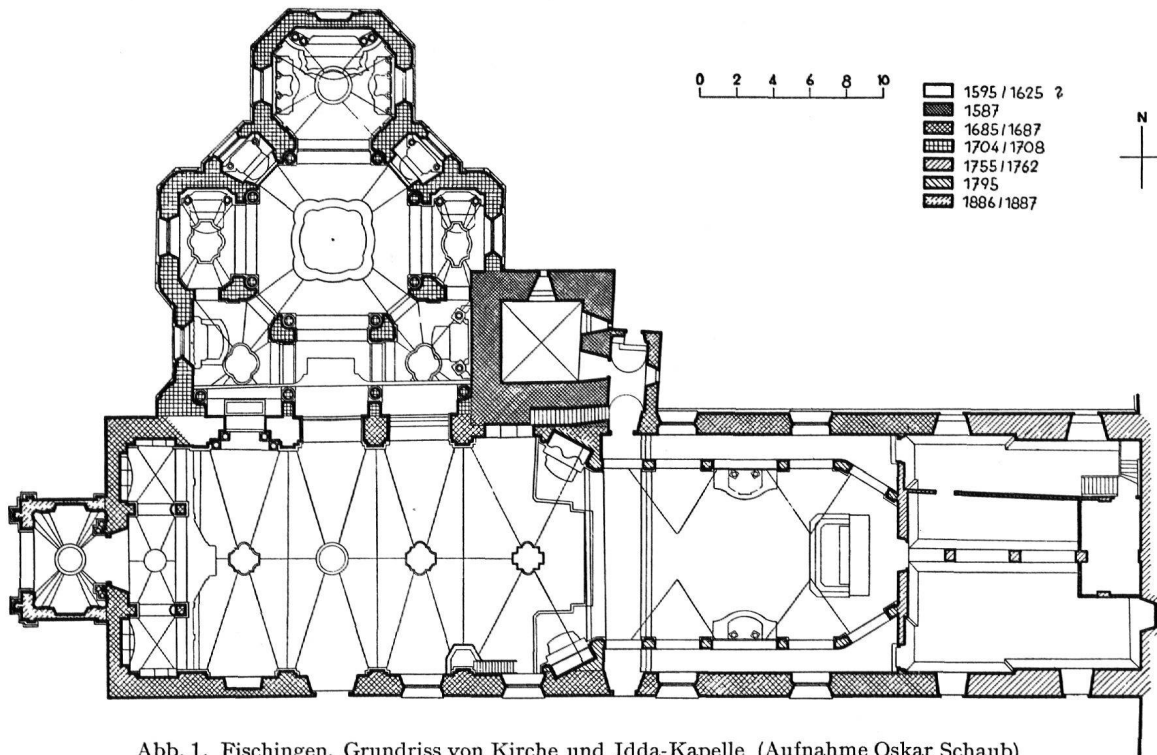
Abb. 1. Fischingen, Grundriss von Kirche und Idda-Kapelle (Aufnahme Oskar Schaub)
