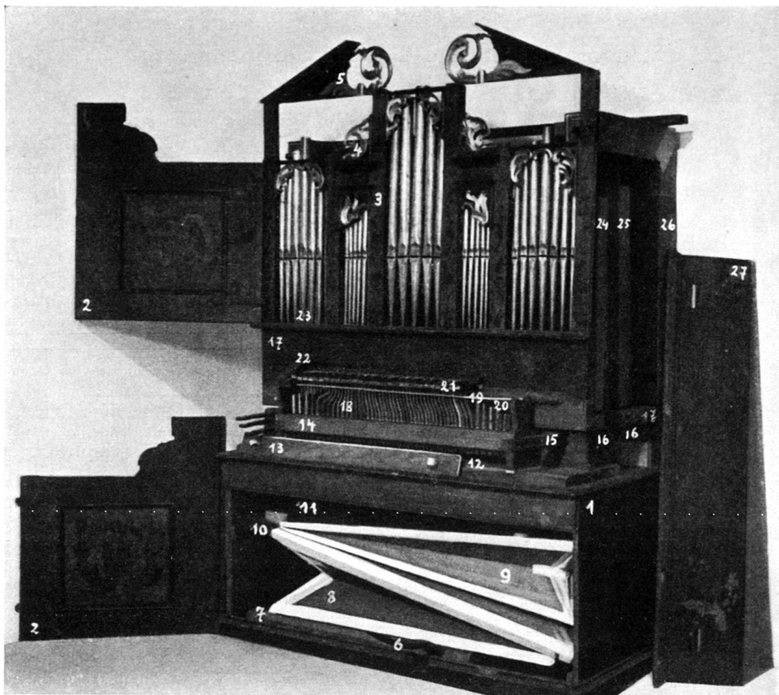
Abb. 12. Fünfteilige Hausorgel Joseph Loosers a. d. J. 1784, ohne Seitenwände, Rückwand, Gebläsekasten-Vorderwand, Decke und Kranz, im Besitz des Verfassers.
