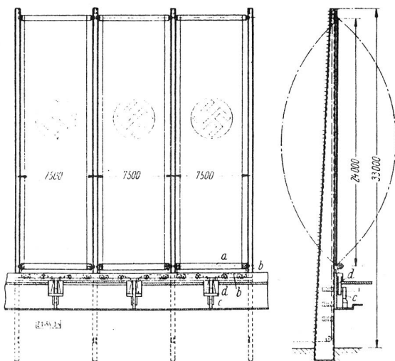
Abb. 4 und 5. Gesamtanordnung der Masten mit Wickelvorrichtung. a Wickeltrommel für das Fahmentuch b Seilzüge mit Kraftübertragung c Windkessel d Druckzylinder
