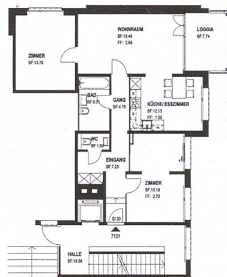
Grundriss einer Dreizimmerwohnung. Bei der Sanierung blieben die Grundrisse unverändert, nur die Eckwohnungen erhielten neu offene Wohnküchen.
