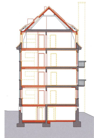
Die baulichen Massnahmen waren so umfangreich, dass die Instandsetzung in unbewohntem Zustand erfolgte. Teils mussten Böden und Decken bis auf die Rohkonstruktionen zurückgebaut werden.
