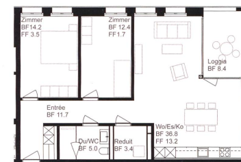
Grundrisse zweier 3 ½-Zimmer-Wohnungstypen.
