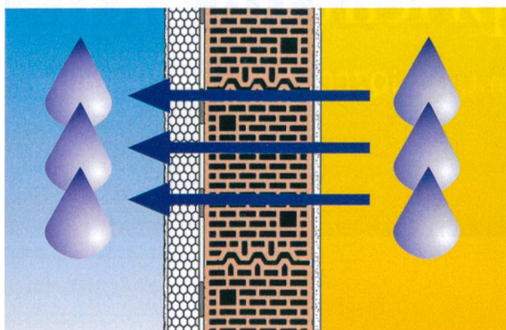
Bis 10 Liter Wasserdampf müssen pro Haushalt und Tag nach aussen dringen. Die Baunit Open-Klimafassade leistet dazu einen wichtigen Beitrag, denn die Fassadenplatte «open Therm» Duo hat den gleichen Diffusionswiderstand wie eine Ziegelwand.
