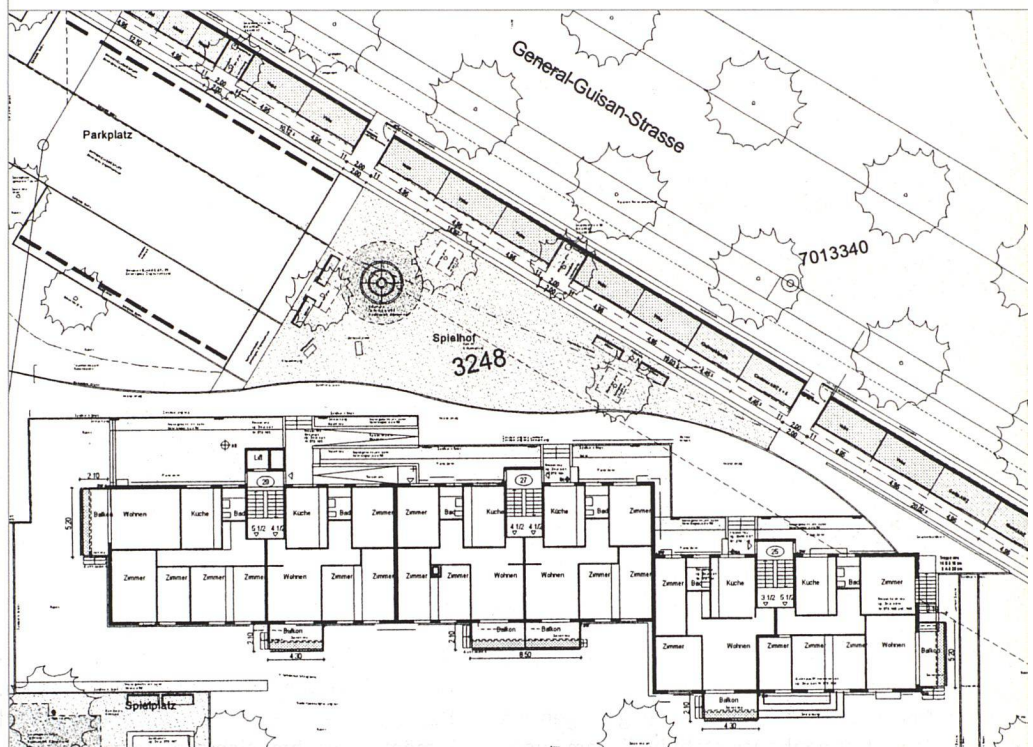
Situationsplan der Siedlung Herti I der Allgemeinen Wohnbaugenossenschaft Zug (AWZ). Im Rahmen einer Neugestaltung der Umgebung entstand entlang der General-Guisan-Strasse ein langgezogener Fahrwand-Unterstand. Einerseits schirmt er die Siedlung gegen den Lärm ab, andererseits ermöglichte er eine Aufwertung des nördlichen Hofbereichs. Vergrösserte Balkone mit Vollverglasung bieten gleichzeitig auf der Südseite mehr Wohnraum.
