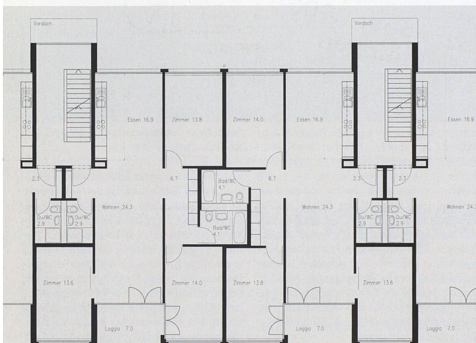
Grundriss Obergeschoss. Bemerkenswert ist der durchgehende Wohn-/Essraum.
