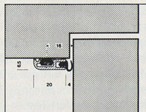
Türsanierung HEBGO 126/634
