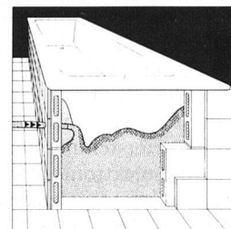
STARTEX in Duschen- und Bade- wannen-Hohlräumen (Gerausch- u. Temperaturabfallverringering).
