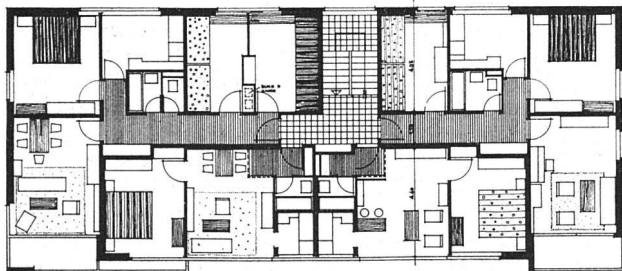
Grundriß Obere Wildeggsstraße
