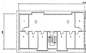
GRUNDRISS DACHGESCHOSS
