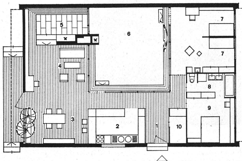
1 Eingang 2 Küche mit Arbeitstisch gegen Hof und Anrichte gegen Eßteil 3/4 Wohn-Eßraum 5 Cheminéeerraum, ebenerdig zum Hof 6 Atriumhof mit Außencheminée 7 Kinderkojen mit gemeinsamem Spielplatz 8 Bad und WC 9 Elternschlafzimmer 10 Abstellraum
