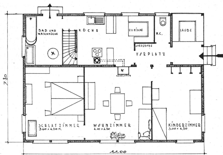
GRUNDRISS.
