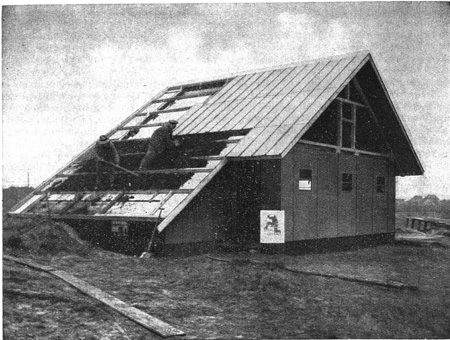
Stahlamellen-Siedlungshaus im Bau
