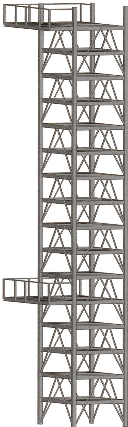
Die Säulenkonstruktion des Turmes. Hier sichtbar gemacht sind die vier Säulen, die Windverbände, die Hori- zontalträger und die Plattformen. Computersimulation: PlanQuadrat AG, Willisau
