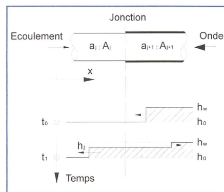
Figure 3. Transition et réflexion d'une onde de pression incidente ( h_w-h_0 ) en traversant une jonction qui sépare deux régions de puits de caractéristiques hydroacoustiques distinctes.
