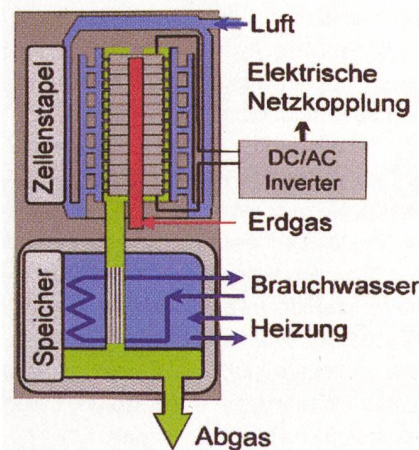
Bild 1. Brennstoffzellenstapel mit integriertem Wärmespeicher.
