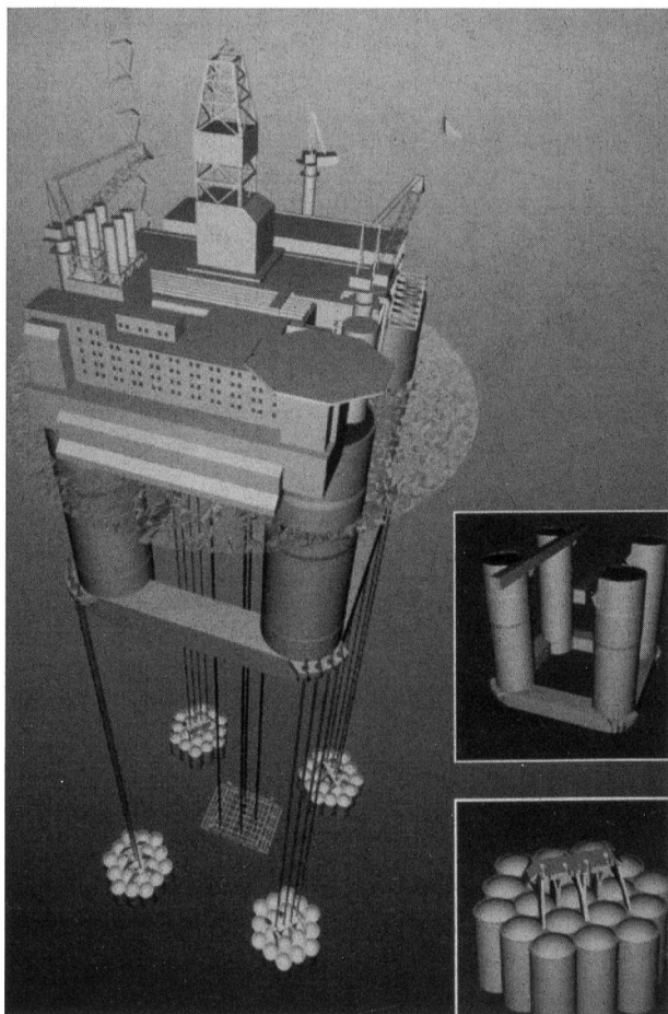
Bild 1. Schwimmende Ölförderplattform (TLP) Heidrun, bestehend aus: Deckskonstruktion (Tosides), Schwimmkörper, Zugbändern (Tension Legs) und Fundamentkonstruktionen.
