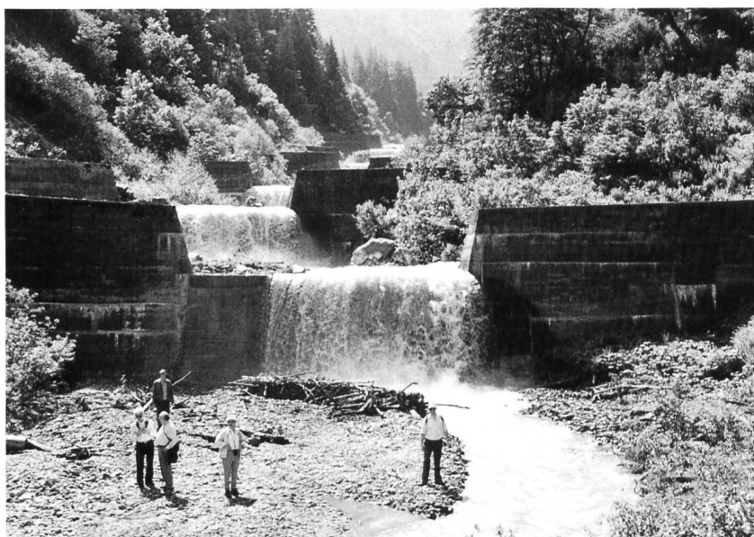
Bild 1, links. Der untere Teil der Sperrentreppe im Durnagelbach hält die Seitenhänge zurzeit gerade so stabil, dass sich die Vegetationsdecke wieder zögernd aufbauen kann.
