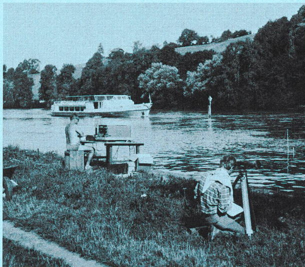
Systematische Wellenmessungen am Fahrgastschiff «Arenenberg», Rhein bei St. Katharinental. Am Ufer links der Tisch mit den elektronischen Mess- und Registriergeräten, rechts das Stativ mit Telemeter zur Distanzmessung.
