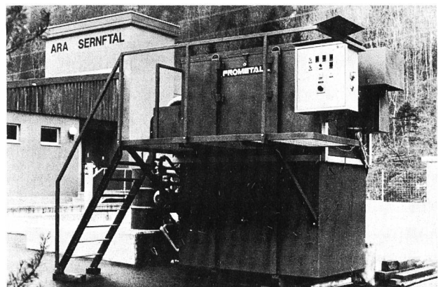
Versuchsanlage in der ARA Serntal der Prometall AG. Biologische Anlage: Tauchtropfkörpersystem. Versuchsfilter: PFU-4 in Stahlwanne (etwa 2000 EGW). Filteroberfläche: 4,8 m 2 . Filterbelastung: etwa 13 m 3 /h. Zulaufkonzentration im Durchschnitt: etwa 20 mg ss/l. Abflusskonzentration Filter: etwa 5 mg ss/l.
