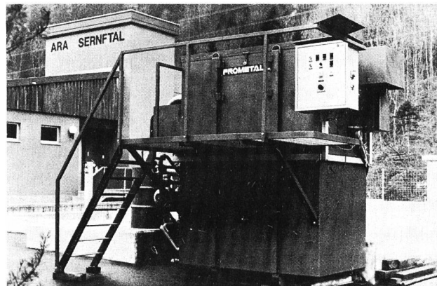
Versuchsanlage in der ARA Sernftal der Prometall AG. Biologische Anlage: Tauchtropfkörpersystem. Versuchsfilter: PFU-4 in Stahlwanne (etwa 2000 EGW). Filteroberfläche: 4,8 m². Filterbelastung: etwa 13 m³/h. Zulaufkonzentration im Durchschnitt: etwa 20 mg ss/l. Abflusskonzentration Filter: etwa 5 mg ss/l.
