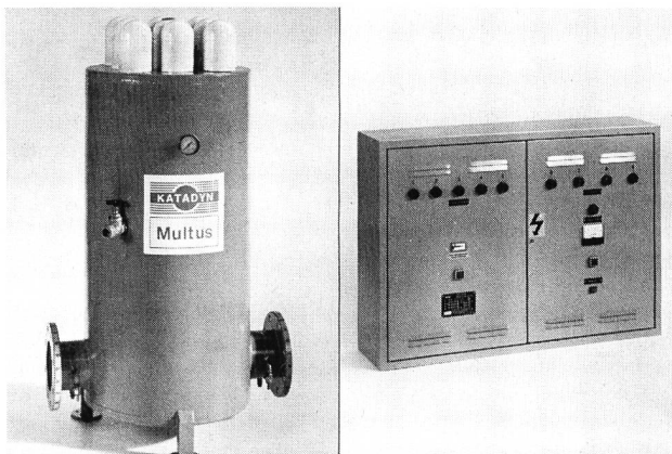
Katadyn Multus UV Kompaktanlage G9 mit einer Leistung bis 120 m³/h.
