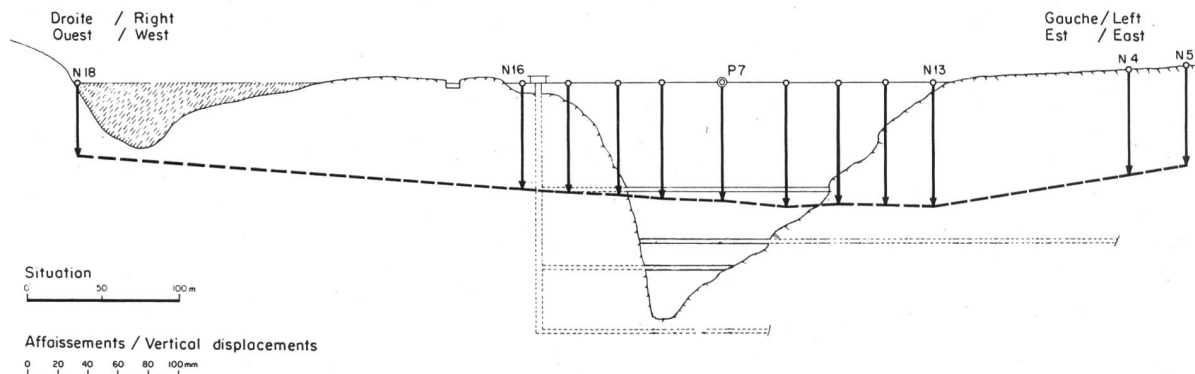
Figure 2. Affaissements entre 1972 et 1979.
