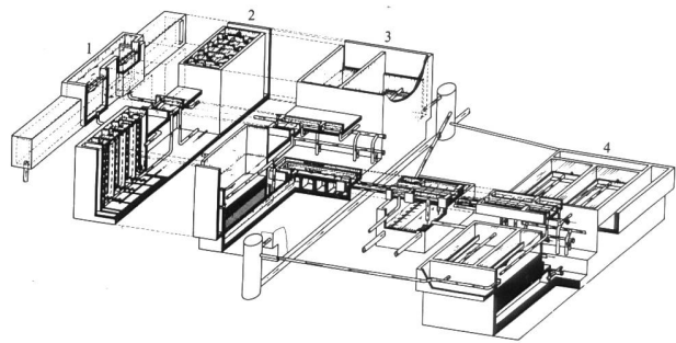
Bild 1. Aufbau der Wasseraufbereitungsanlage Egau (Landeswasserversorgung Stuttgart). 1 Rohwasserrinne, 2 Ozonkontaktkammern, 3 Zweischichtfilter, 4 Aktivkohlefilter.
