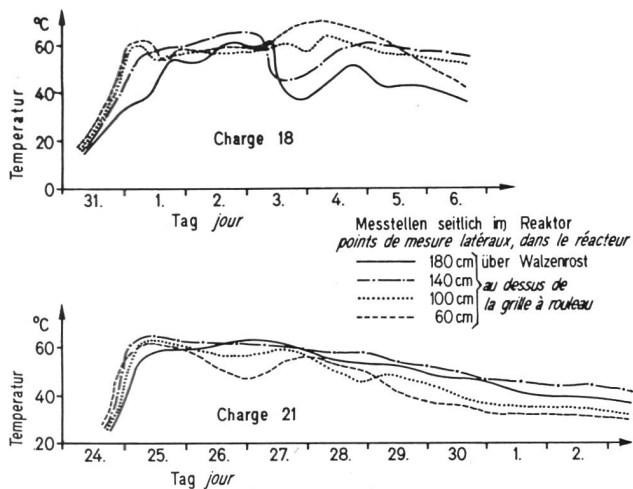
Figure 1. Déroulement de la température dans le réacteur. Au cours de l'intensif processus de décomposition aérobie-thermophile, des températures élevées surgissent dans le réacteur aéré. Du fait que le contenu de réacteur est plusieurs fois remué et retourné par jour, le matériel traverse plusieurs fois les zones chaudes et est parfaitement hygiénisé.
