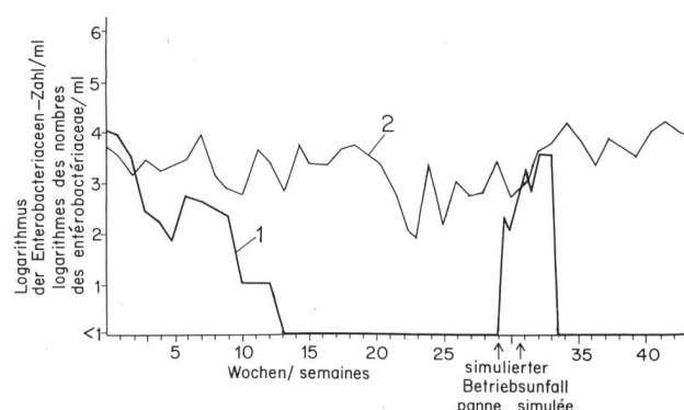
Figure 2. Variation du nombre des entérobactériacées dans les postdigesteurs.
