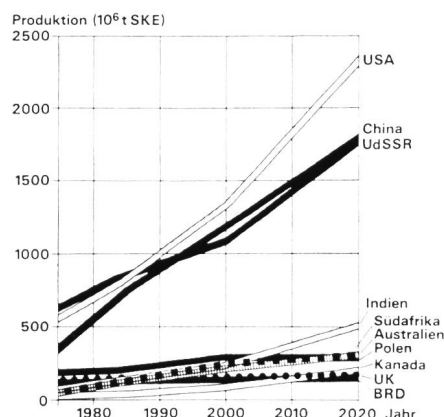
Bilder 11 und 12. Entwicklung der Kohleproduktion.
