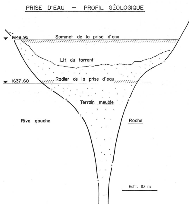
Fig. 10 Aménagement GWK III; prise d'eau, profil géologique.
