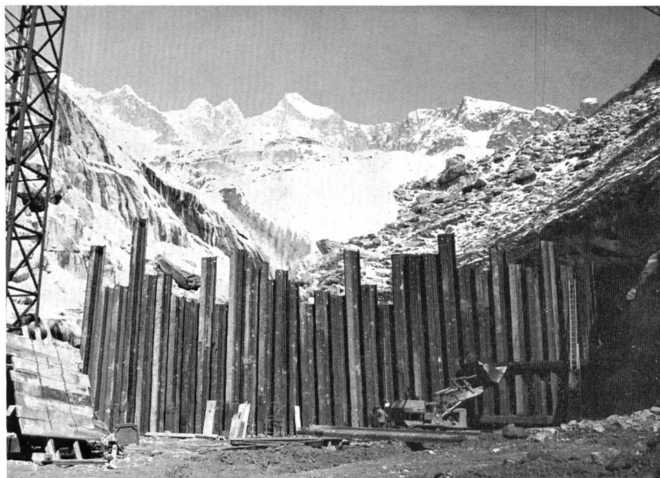
Fig. 1 Forces Motrices de Conches S.A./Gommerkraft- werke AG: GKW III Chantier de la prise d'eau près du glacier de Fiesch; rideau de palplanches.
