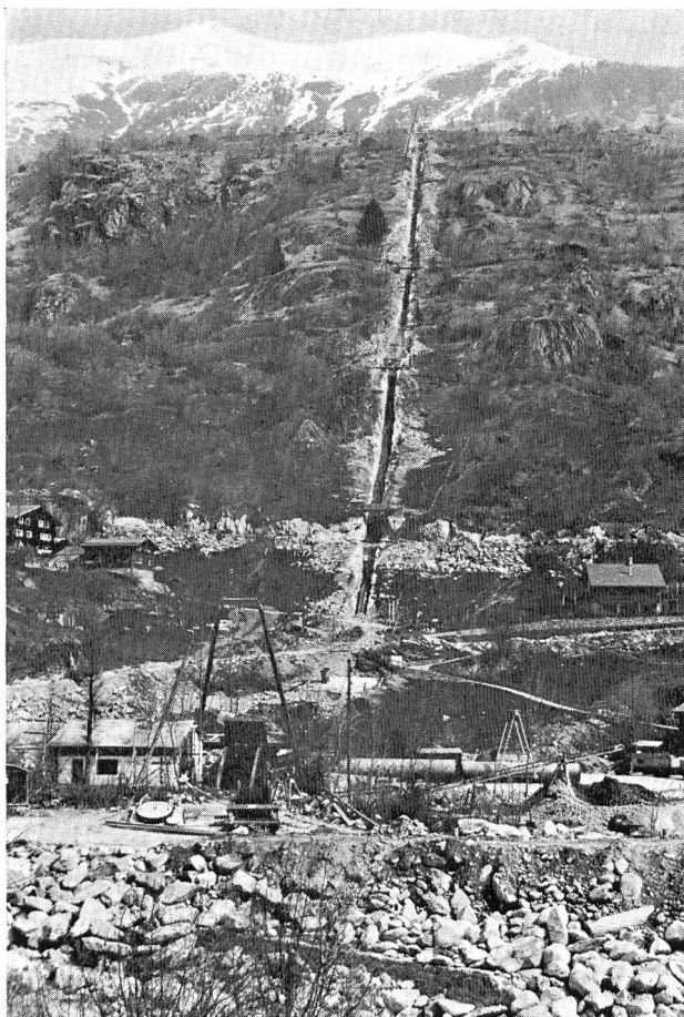
Fig. 12 Aménagement GKW III; chantier de la conduite forcée.
