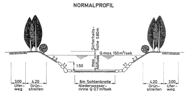
Bild 4 Normalprofil — Fischerei, mit Niederwasserrinne bei ungenügender Abflusstiefe.
