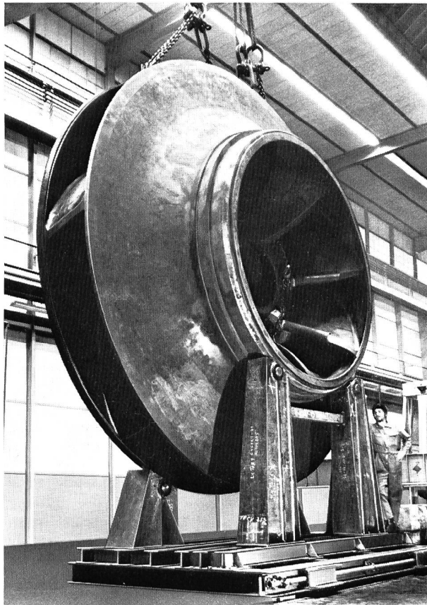
Das Bild zeigt das Laufrad der Pumpenturbine, das für das Kraftwerk Voglans (Ain) der EdF bestimmt ist. Dies ist die grösste Pumpenturbine Europas und die erste in Frankreich. Es ist eine franko-schweizerische Verwirklichung, zu der die ACMV einen grossen Teil beigetragen hat.
