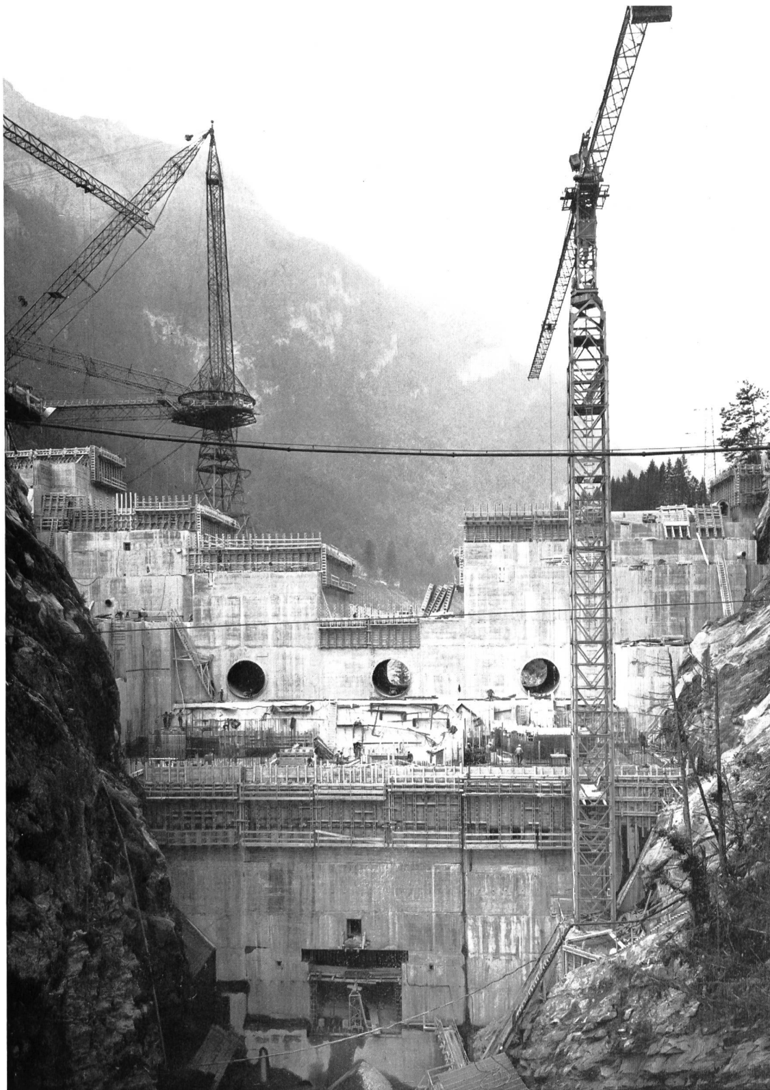
Luftseitige Ansicht der Staumauer Mapragg mit vorgelagertem Unterbau der Zentrale (Bild 6 des nachfolgenden Berichts).
