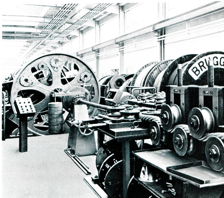
Bild 2 Teilbild aus dem Rundgang durch die Fabrikanlagen der Kabelwerke Brugg.
