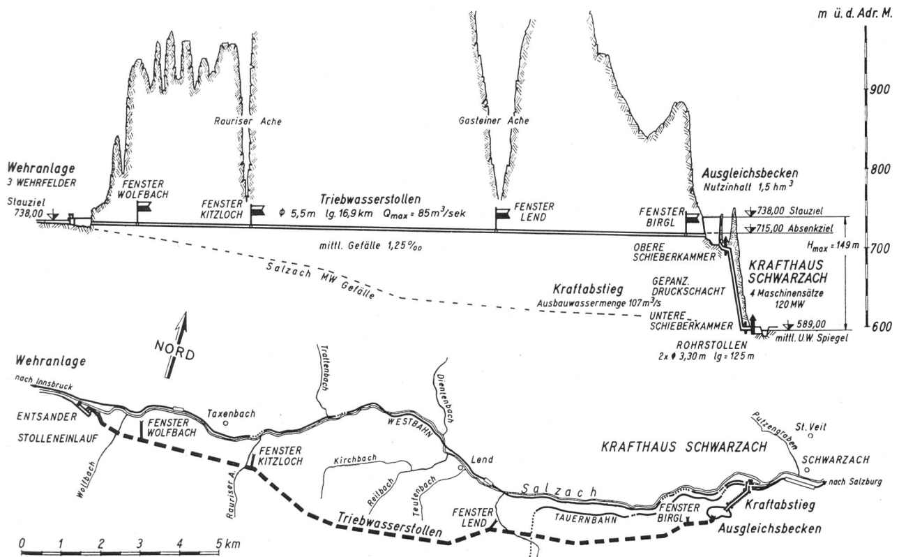
Bild 1 Längenprofil und Lageplan des Kraftwerkes Schwarzach
