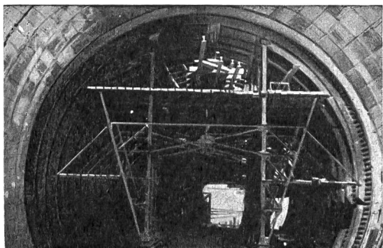
FIX-Stahlschalung
