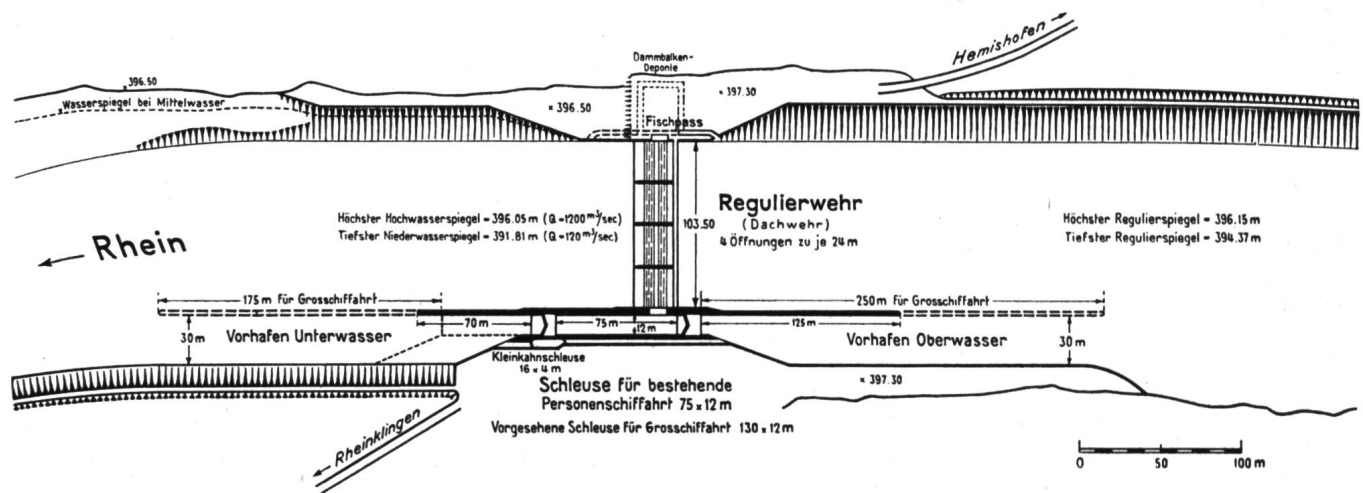
Abb. 3 Situationsplan des Regulierwehres und der Schiffsanagen.
