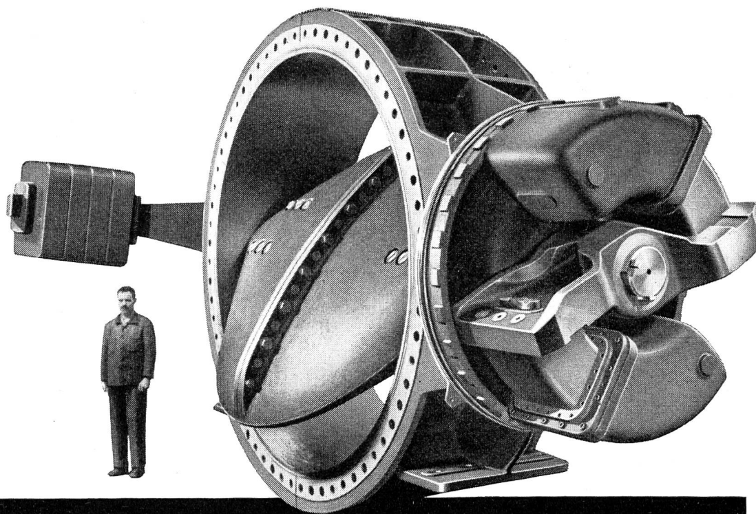
2700 mm Drosselklappe für 10 at Betriebsdruck, mit doppelwirkendem Ringkolbenantrieb und zusätzlichem Hilfs-Schließgewicht.
