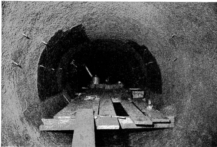
Baustelle Leggistein: Sika-4a-Abdichtung auf wasserführendem Beton.
