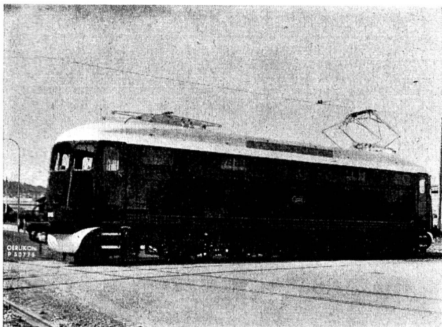
Fig. 15 Ansicht der 1-Do-1-Gleichstrom-Lokomotive für die Niederländischen Eisenbahnen.
