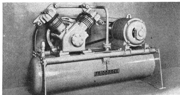
Fig. 13 Frigorrex-Kühlaggregat VJW.
