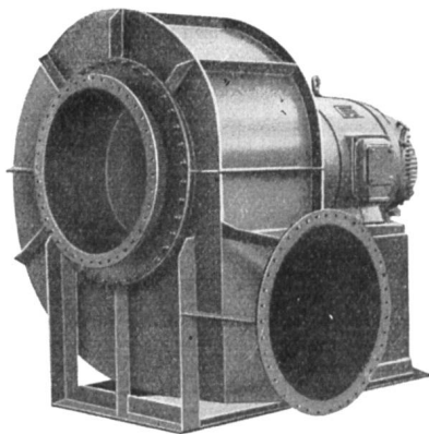
Fig. 19 Ventilator in gasdichter Ausführung für 2 Atü Ueberdruck.
