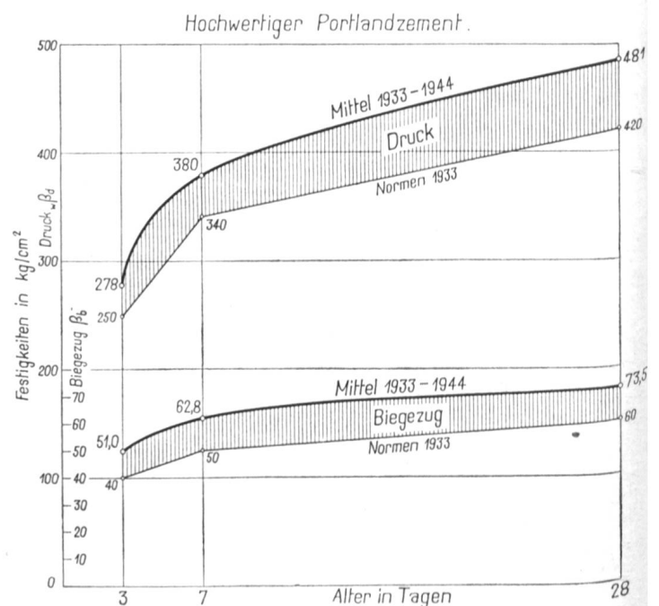
Abb. 6 Schweizerische hochwertigste Portlandzemente (HPZ) 1933 bis 1944. Gesamt-mittelwerte der Biegezug- und Würfel-druckfestigkeiten. Alter 3, 7 und 28 Tage. Normenwerte 1933.
