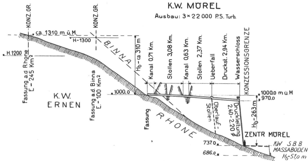
Abb. 2 Kraftwerk Mörel, Längsprofil, Maßstab: Längen 1:250000, Höhen 1:12500. (Nr. 6398 BRB 3. 10. 39.)
