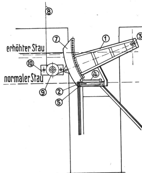
Abb. 3 Segment-Schützenaufsatz (Legende siehe Text).
